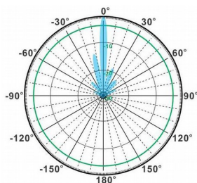
H-Plane
